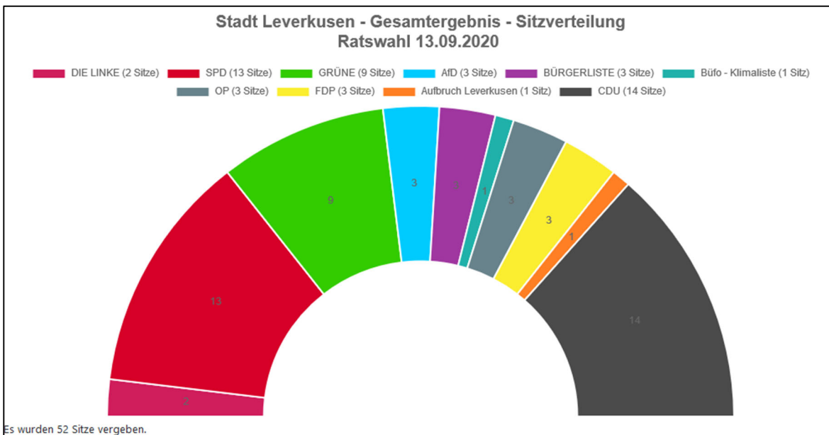
Abbildung 27: Sitzverteilung - Ratswahl 2020
