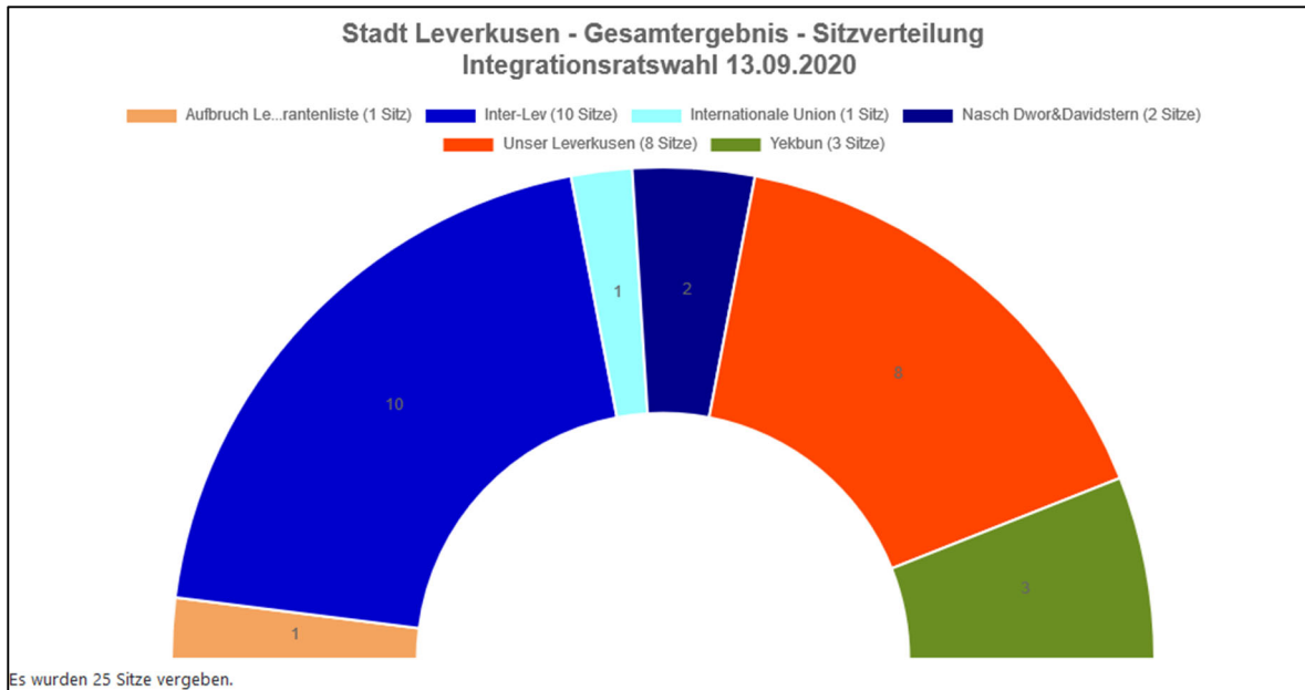
Abbildung 31: Sitzverteilung Integrationsratswahl 2020
