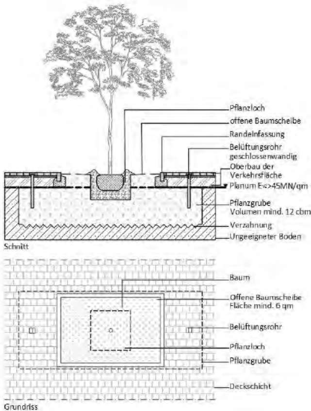
Abbildung 1: Pflanzung in befestigten Flächen; beispielhafte Abbildung, finale Grafik erfolgt analog zum Gestaltungshandbuch; Quelle: Stadt Aachen
