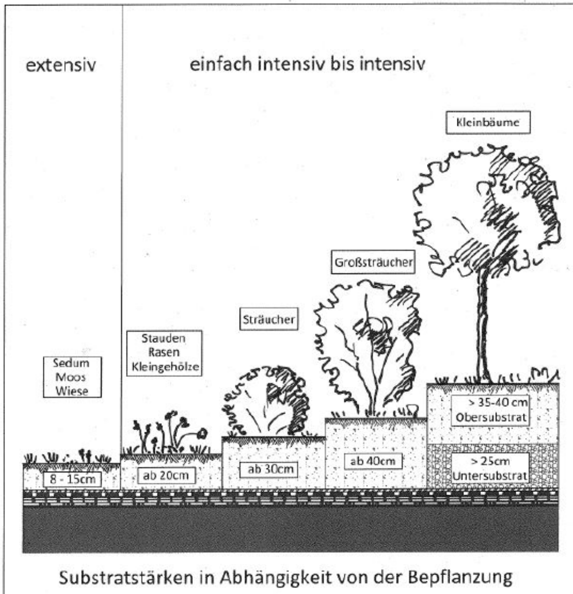
Abbildung 3: Substratstärken Dachbegrünung in Abhängigkeit von der Bepflanzung; beispielhafte Abbildung, finale Grafik erfolgt analog zum Gestaltungshandbuch; Quelle: Stadt Aachen
